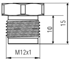
3x M12 Protective cap LAN Port
